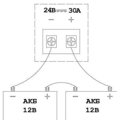
Рис. 3.1.2 Схема подключения АКБ к LPA-DUO
