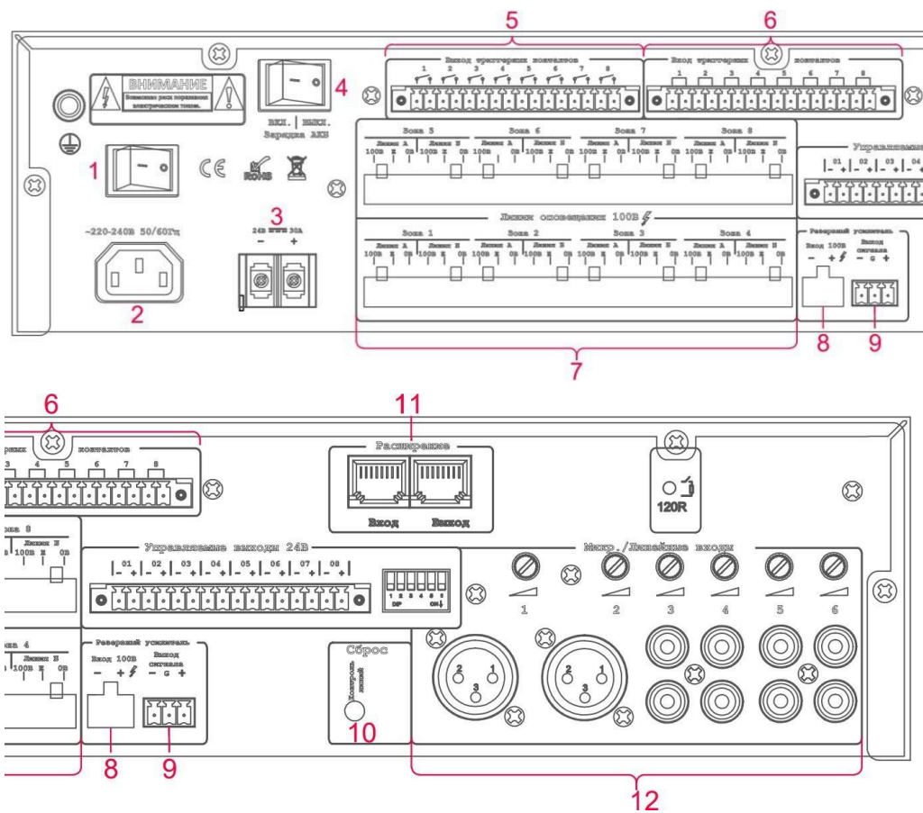
Рис. 2.2.3. Блок расширения LPA-DUO-S (задняя панель)
