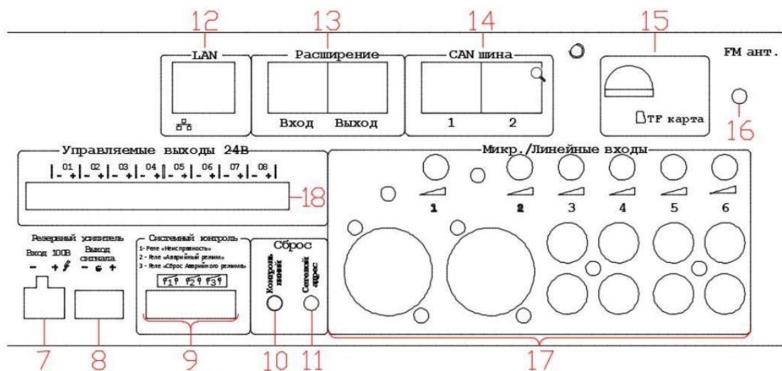
Рис. 2.1.3. Контроллер системы LPA-DUO-M (задняя панель)
